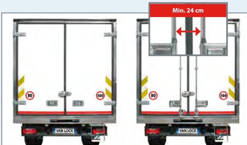
Veicoli dotati di 1 o 2 aste di chiusura, sia interne che esterne Vehicles equipped with 1 or 2 lock-bolts (internal and external)
