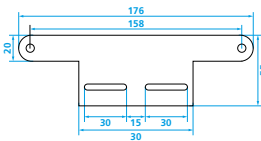
SUPPORTO PER CATARIFRANGENTE TARGA In alluminio anodizzato. Asole di fissaggio.
